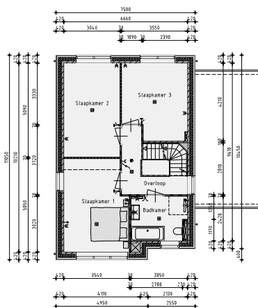
1ste Verdieping
