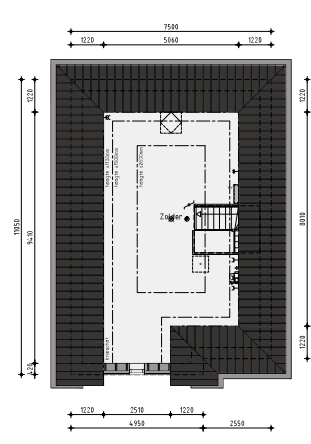
2de Verdieping
