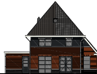
Achtergevel
