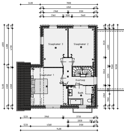
1ste Verdieping
