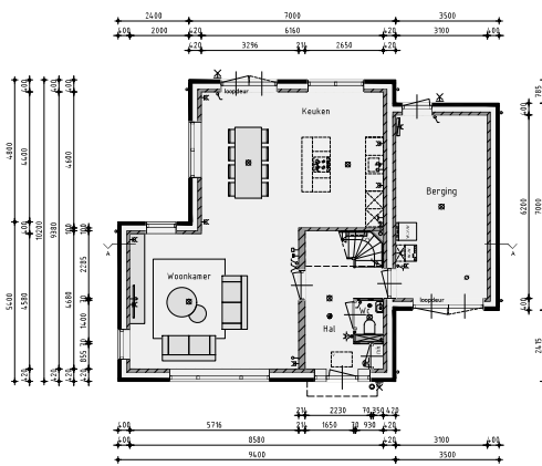
Begane grond
