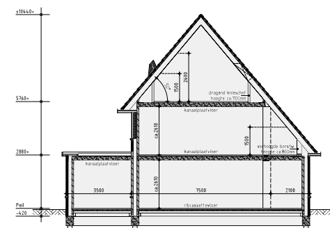
Principe doorsnede A-A
