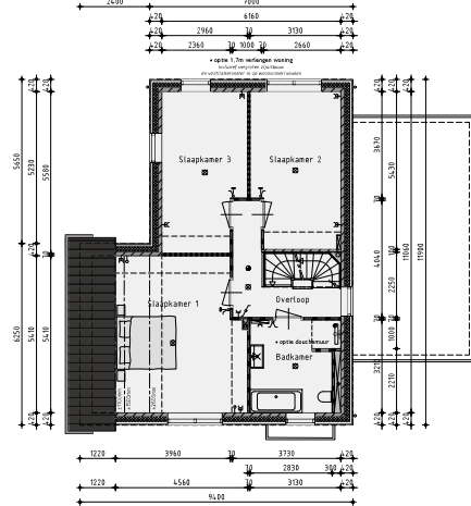
1ste Verdieping
