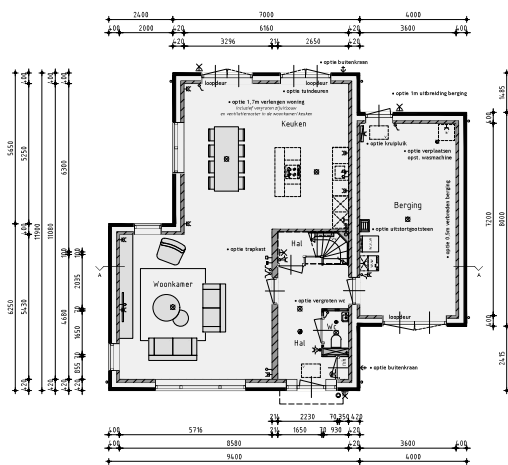
Begane grond
