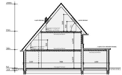
Principe doorsnede A-A
