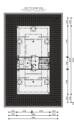
2de Verdieping
