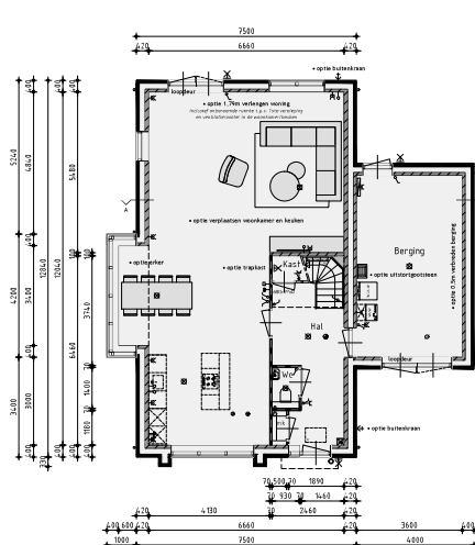
Begane grond
