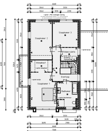
1ste Verdieping
