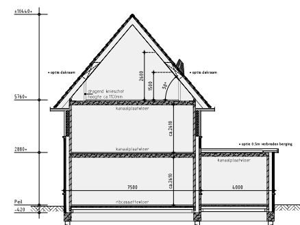
Principe doorsnede A-A
